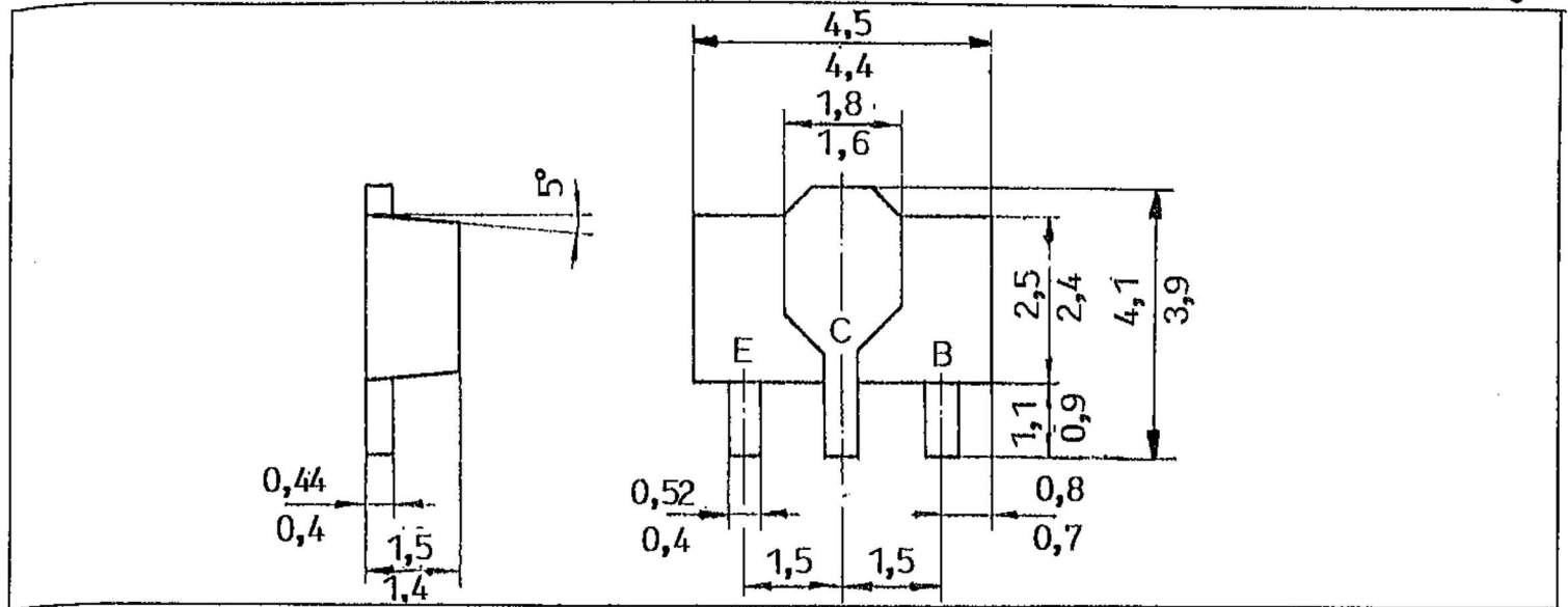
Maßbild mit Anschlußbelegung
