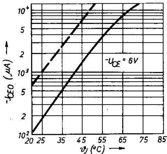
Emitter-Reststrom als Funktion der Sperrschichttemperatur
