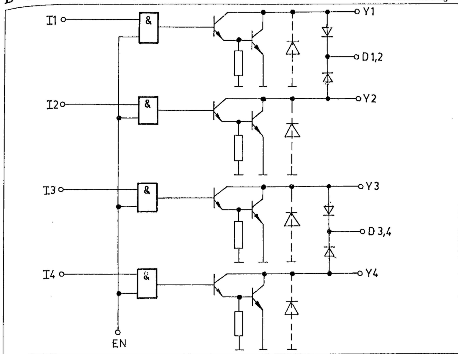
Übersichtsschaltplan
